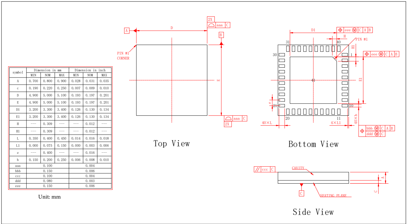
图 7-2. LGA40 (5x5 mm) 封装
