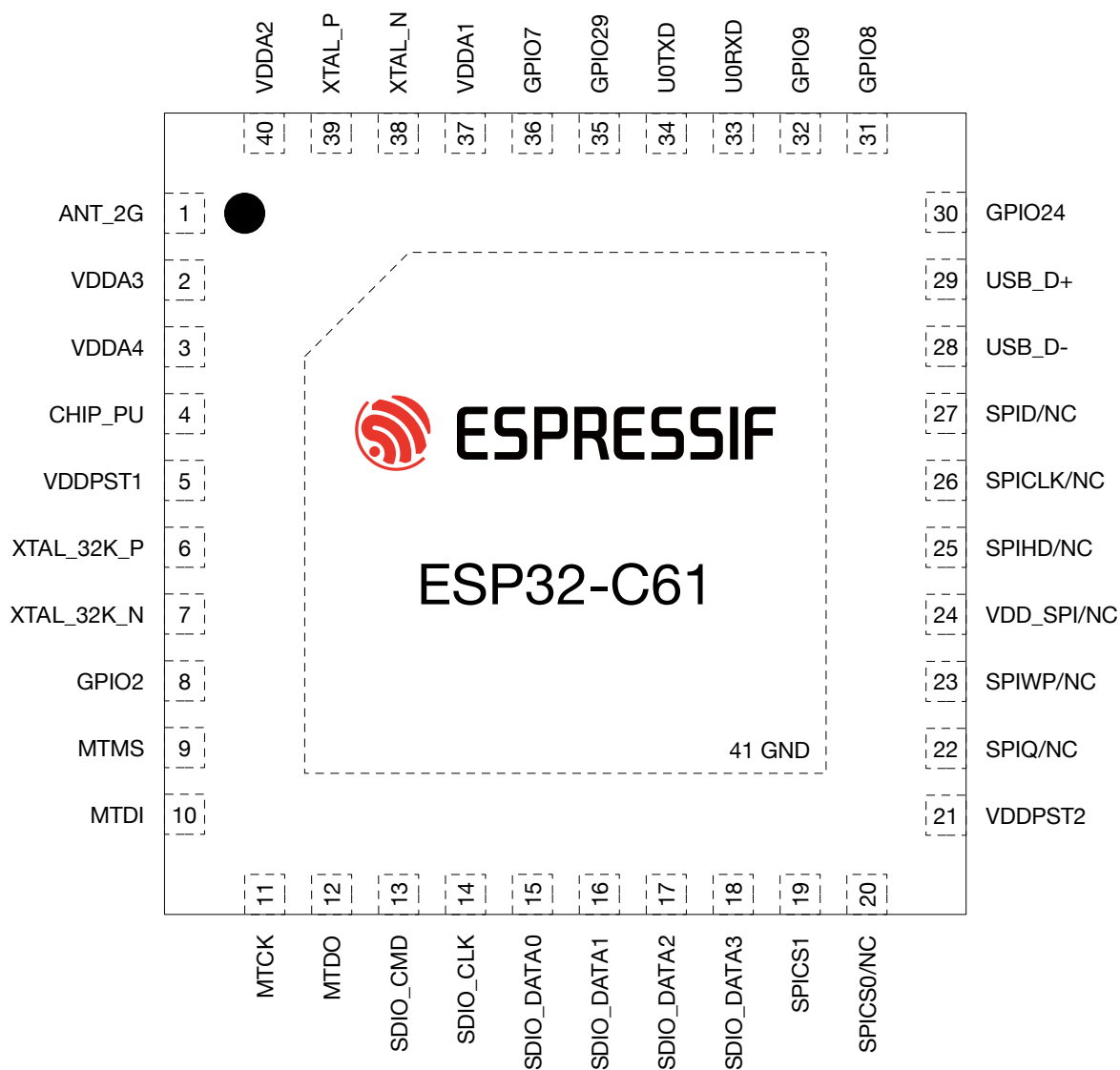
图 2-1. ESP32-C61HR2 & ESP32-C61HR8 & ESP32-C61HF4 管脚布局 (俯视图)
