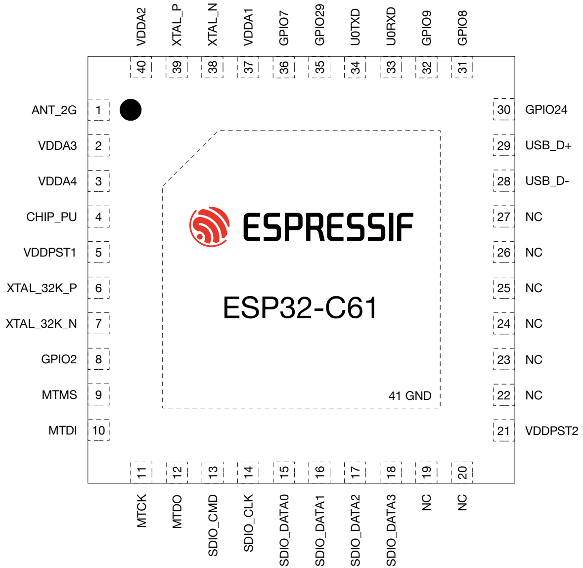
图 2-2. ESP32-C61NF8R8LA 管脚布局 (俯视图)
