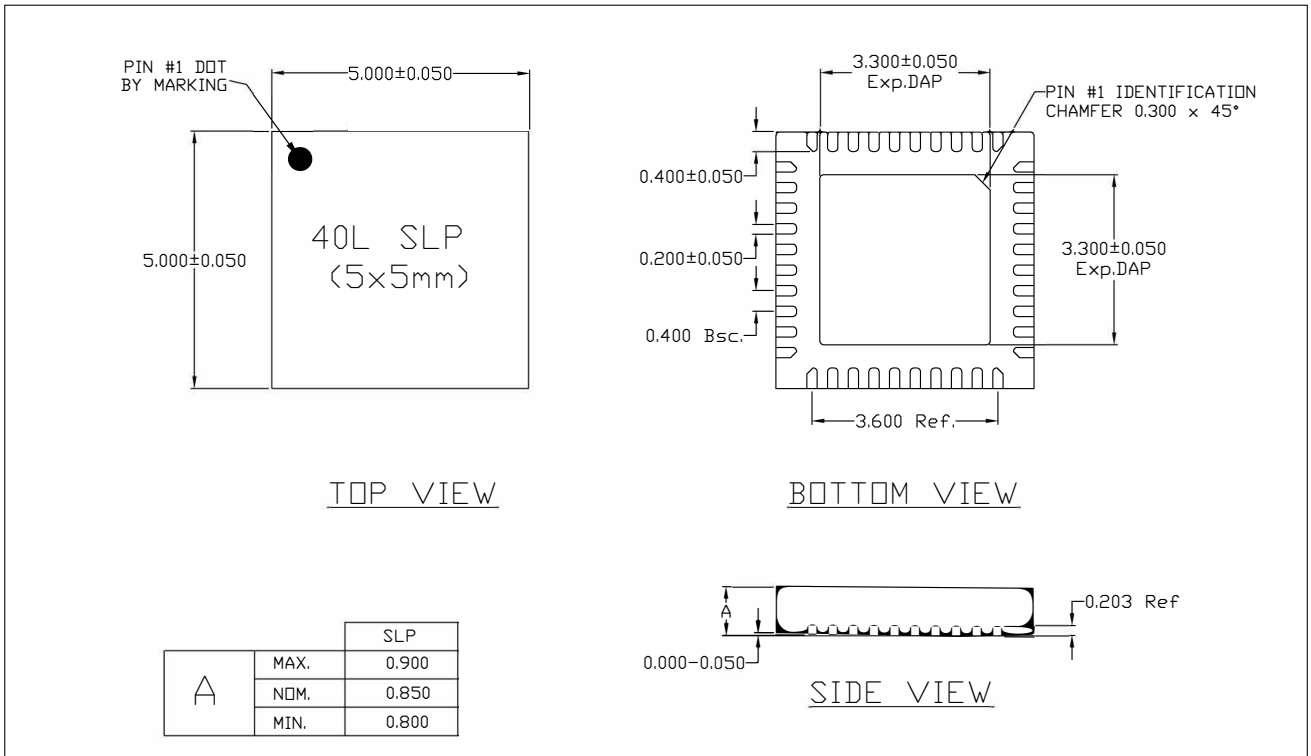
图 7-1. QFN40 (5x5 mm) 封装
