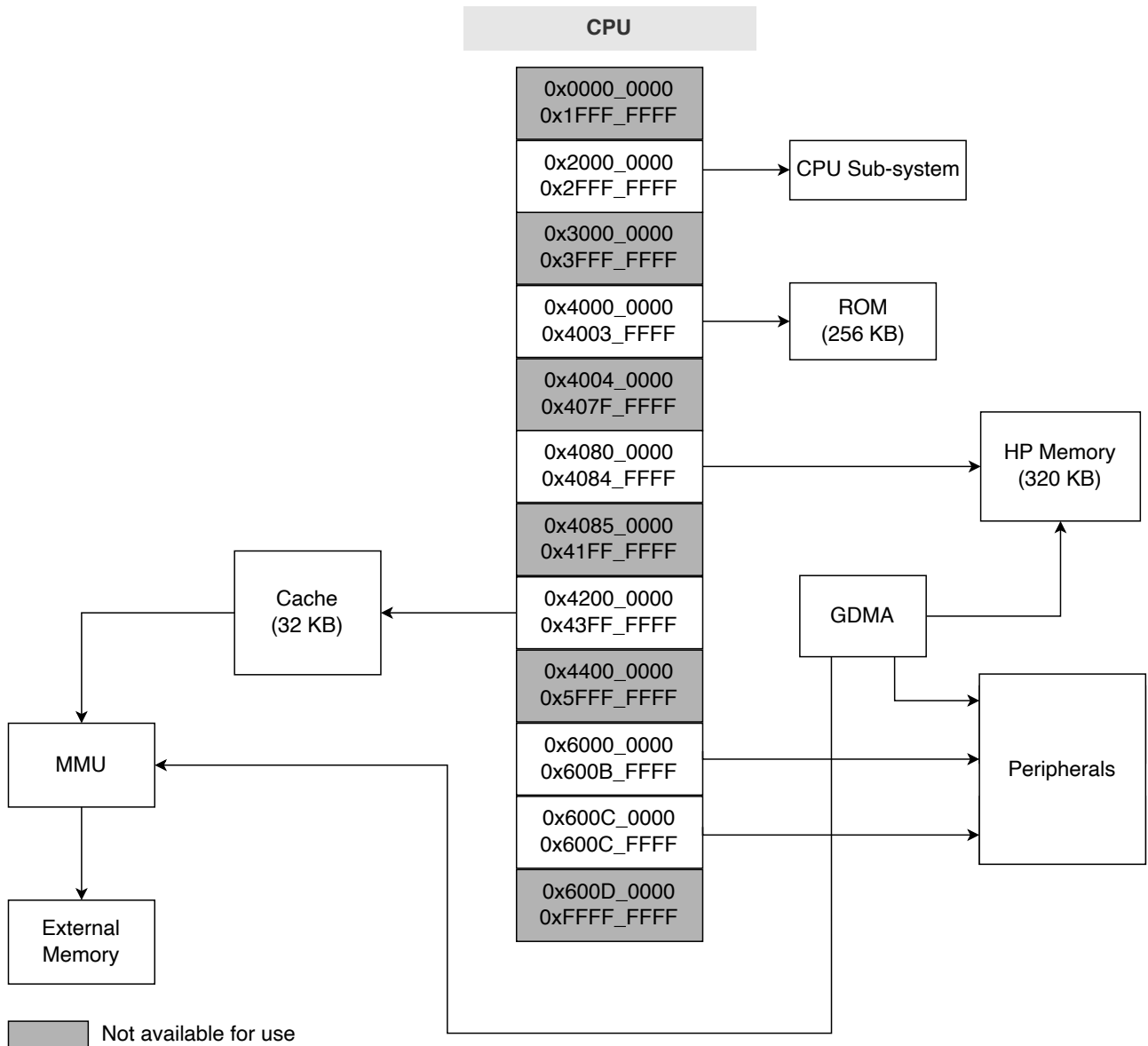
图 4-1. 地址映射结构
