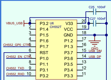
CH552
