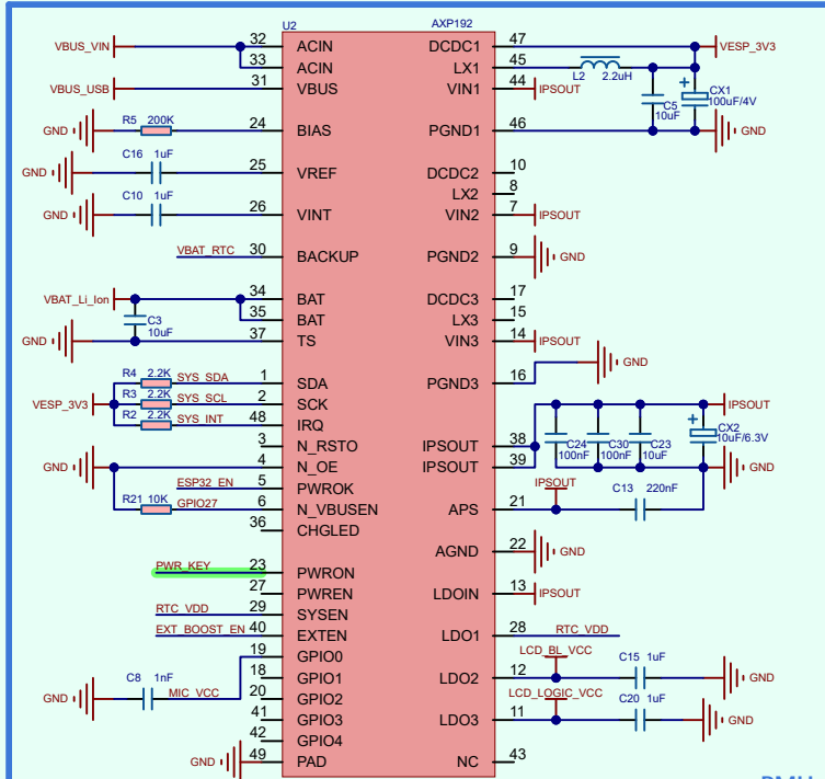
PMU
