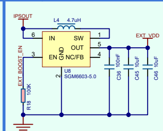
5VOUT_BOOST
