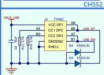
USB TYPE-C
