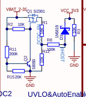
UVLO&AutoEnable
